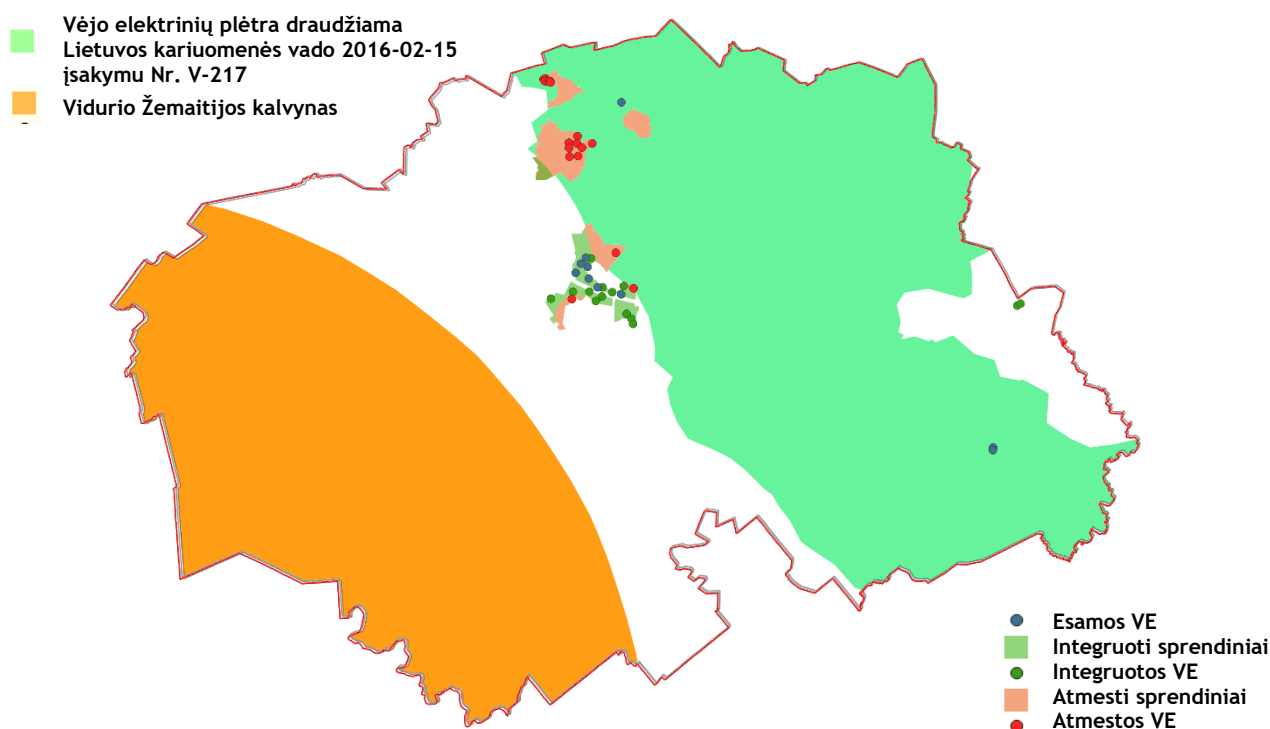
Pav. 6 Patvirtintų saulės ir vėjo energetikos specialiųjų planų sprendinių integravimo statusas
