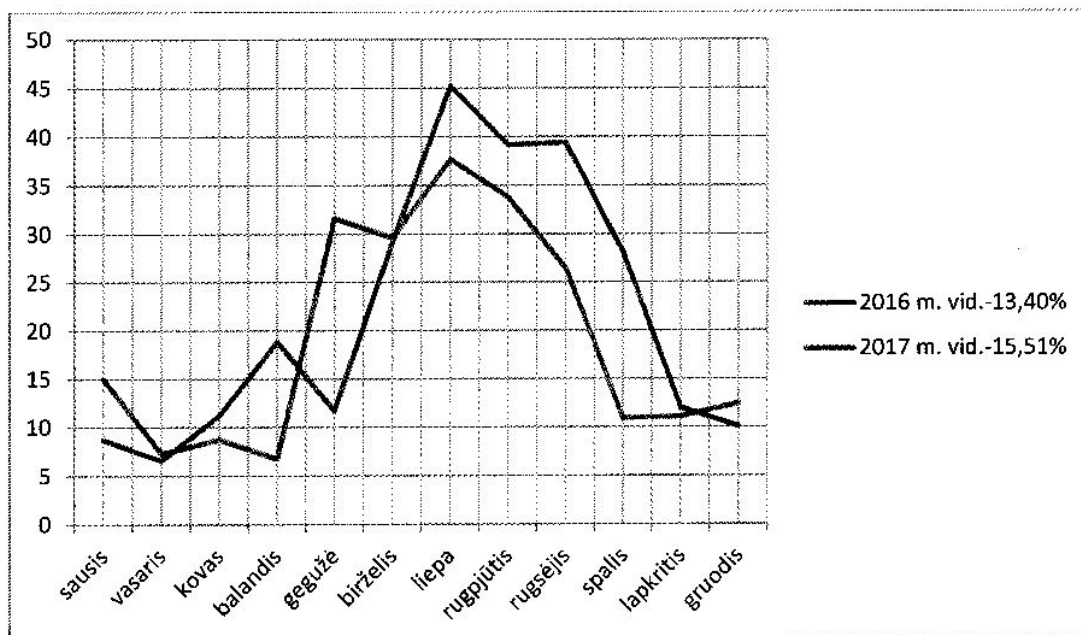
2016-2017m. nuostolių tinkluose (procentine išraiška) palyginimų diagrama :
