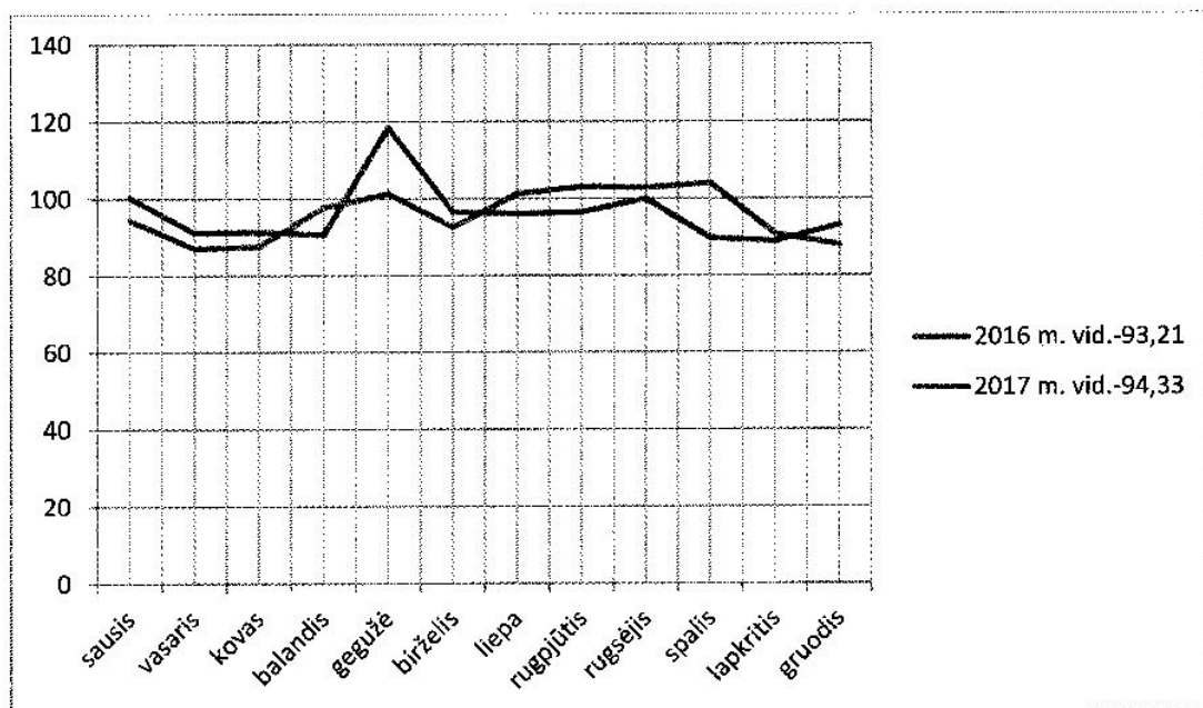
2016-2017m. sunaudoto biokuro (kg/1MWh) palyginimų diagrama :
