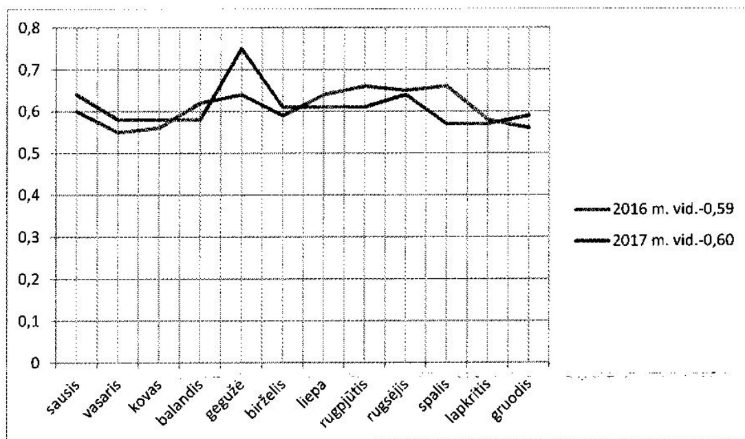
2016-2017m. sunaudoto biokuro (ktm/1MWh) palyginimų diagrama :
