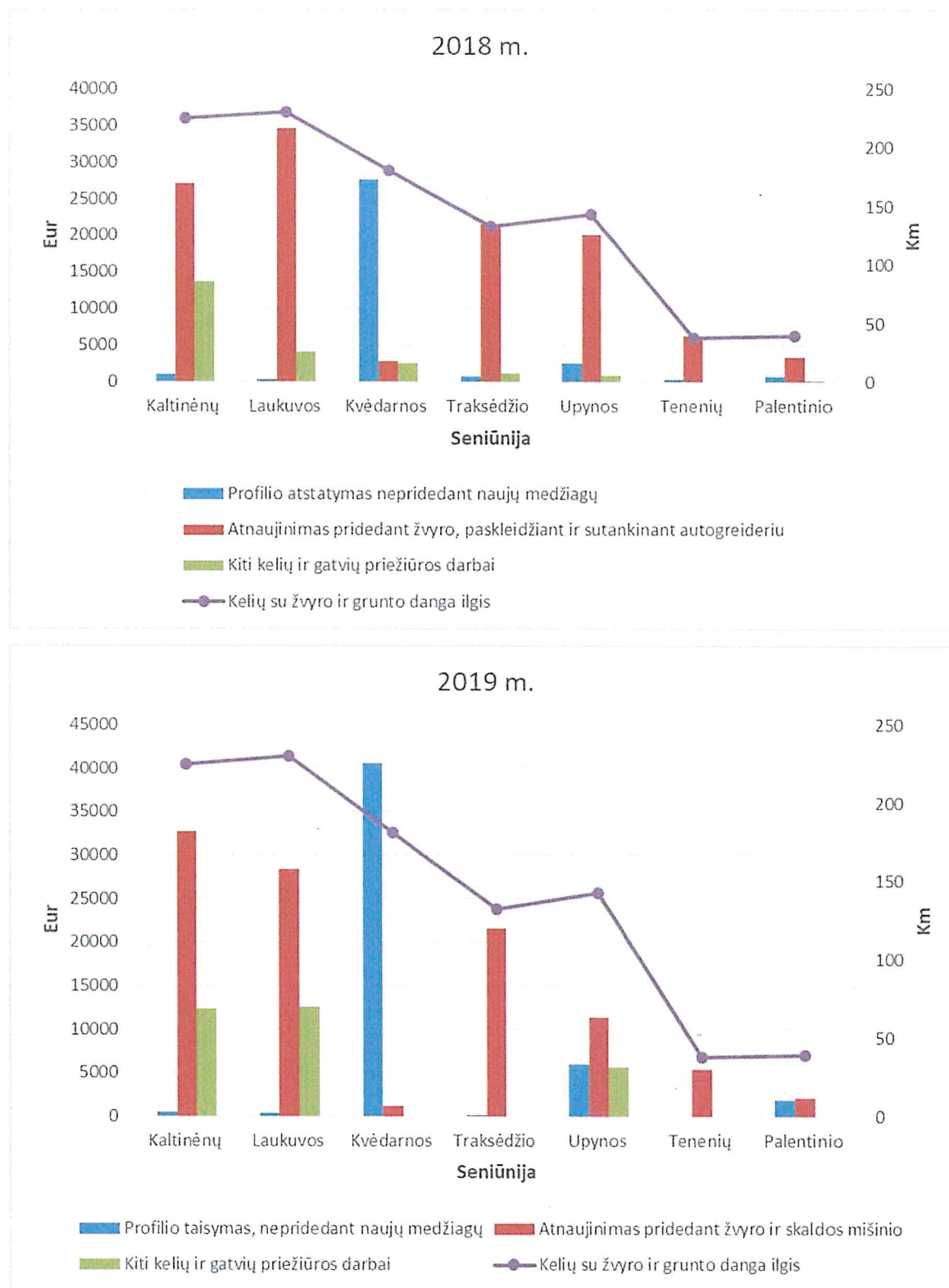
5 pav. Kelių (gatvių) su žvyro ir grunto danga priežiūros darbai seniūnijose 2018 ir 2019 m.
